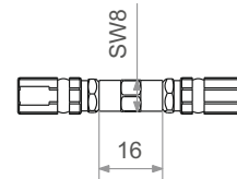
Kupplung Vario
